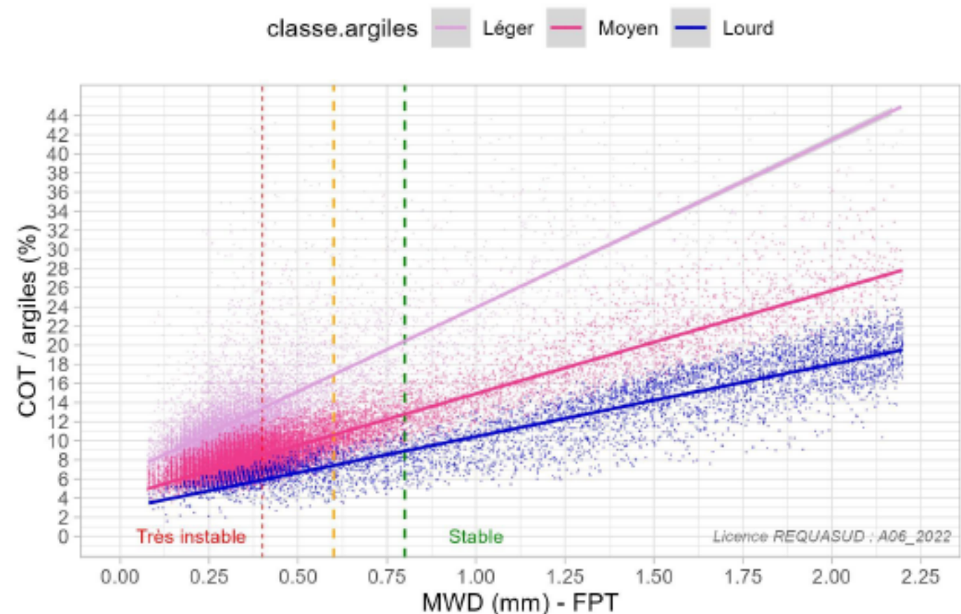
Figure 3.3 : relation entre MWD estimé (Mean Weight Diameter - mm) des agrégats et indicateur COT / argiles issu de l'analyse de données de la BDsol de Requasud (licence A06/2022) et de la carte 'corrigée' des teneurs en argiles.
